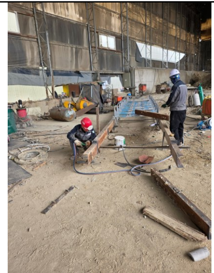
기존설비 철거
