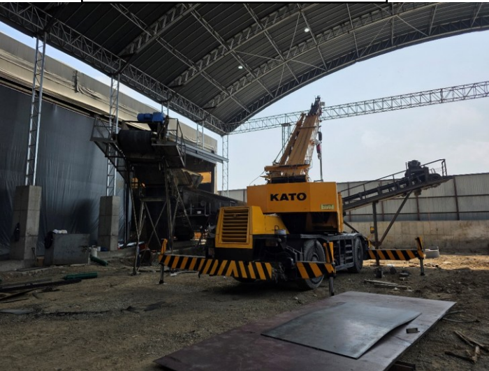
컨베이어설치
